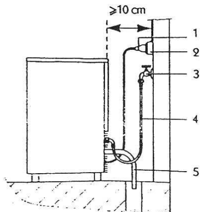
ДИАГРАММА ПОДКЛЮЧЕНИЯ (рис.4)
