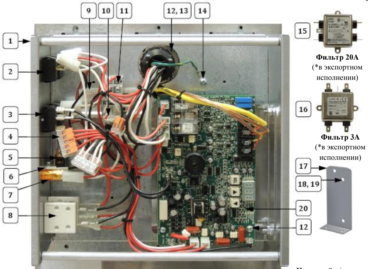
Вид внутренней части блока управления
