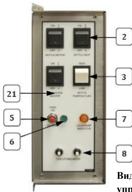
Вид внутренней части блока управления
