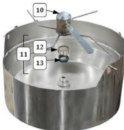
9 Привод мешалки в сборе (включая детали 10 – 14)
