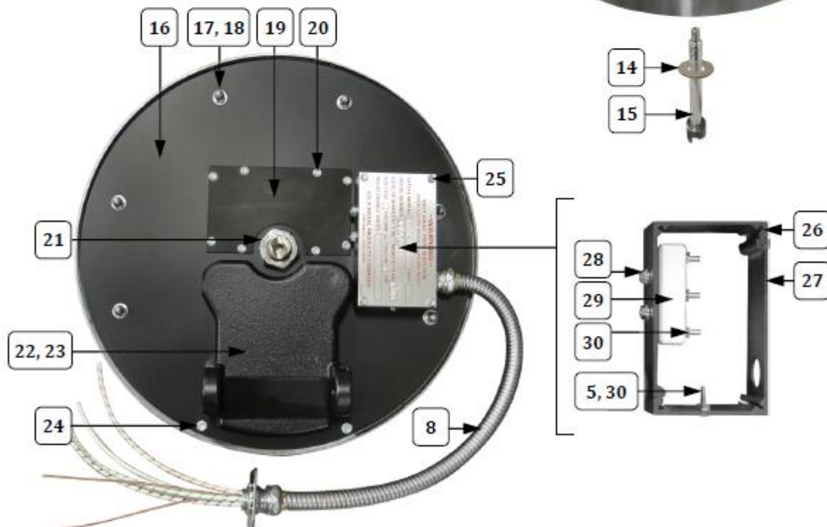
Вид нижней части котла/ распределительной коробки
