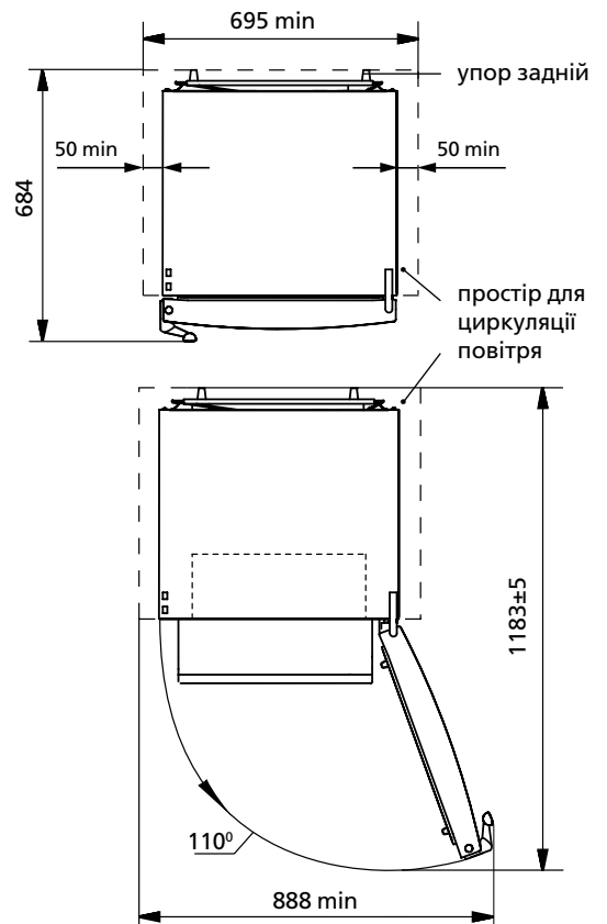
Рисунок 2 – Морозильник (вигляд зверху)
