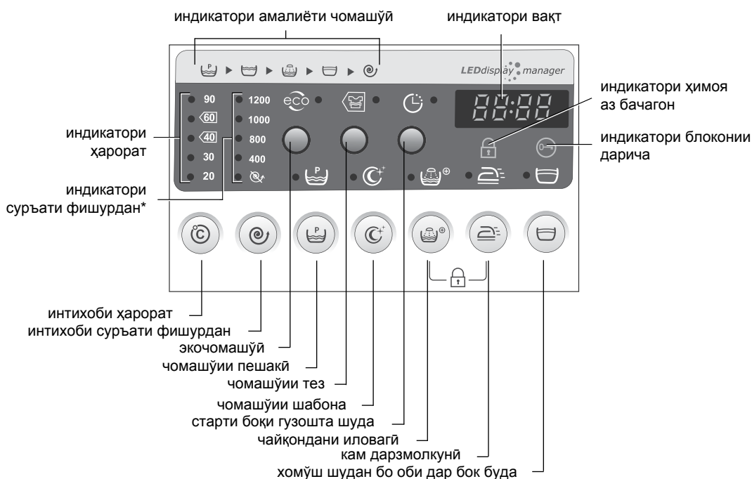
Расми 3 — Зо́наҳои индикатсия ва тугмаҳои интиҳобифунксияҳои иловагӣ
