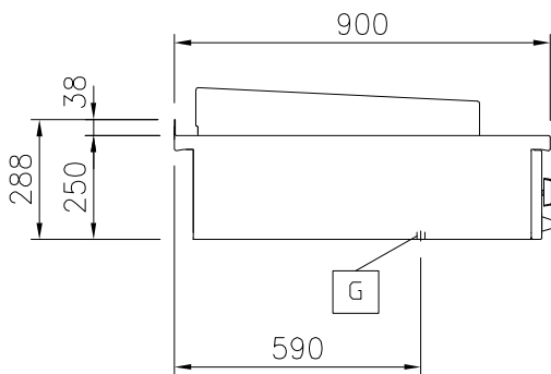
Вид сбоку
