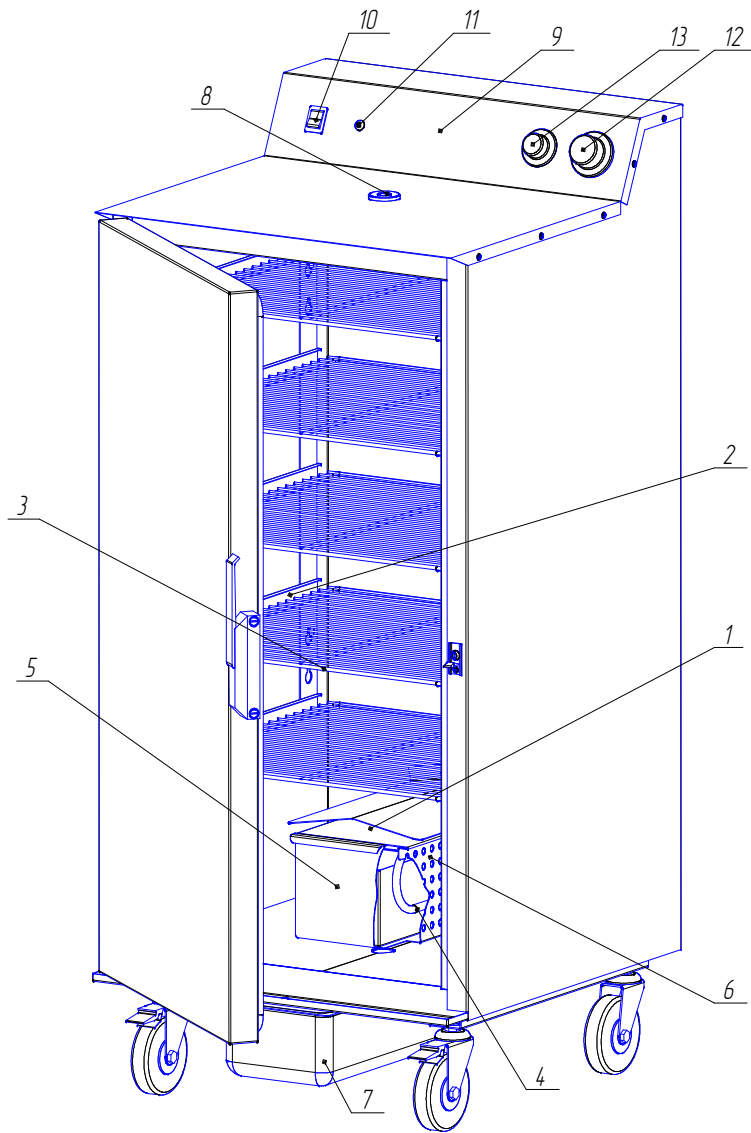
Приложение 1 (Общий вид печи для копчения)
