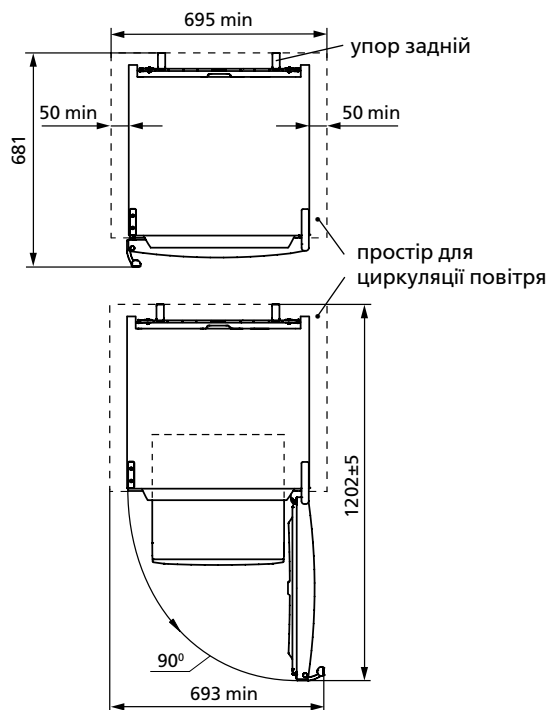
Рисунок 2 – Холодильник (вигляд зверху)
