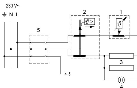
Електросхема
