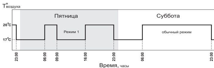
Рис.8 График температуры воздуха в помещении для Режим 3
