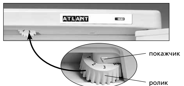
Рисунок 3 – Регулювання температури
