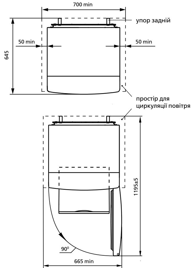
Рисунок 2 – Холодильник (вигляд зверху)
