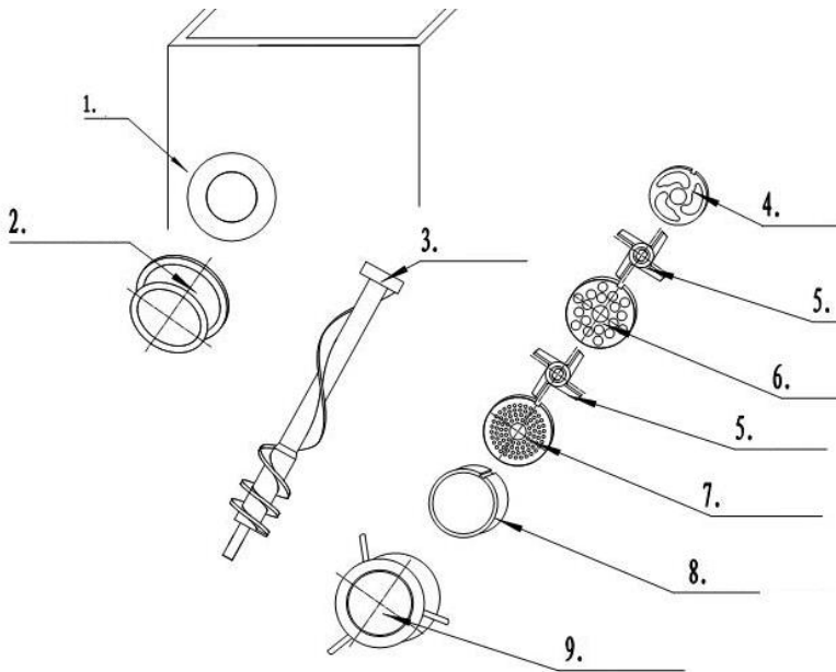
Рис1 Комплектация режущего устройства
