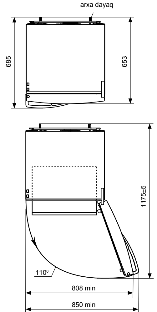
Şəkil 2 – Soyuducu (üstən görünüş)
