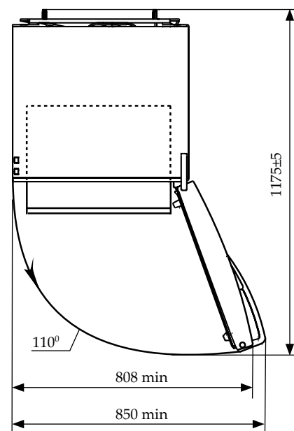
Расми 2 – Яхдон (намуд аз боло)
