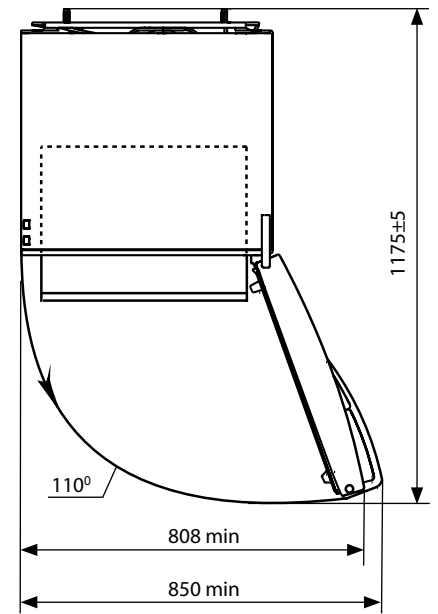
Desen 2 – Frigider (imaginea de sus)
