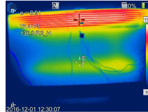
Wild Wind Перегрев 130.9°C на выходе воздуха
