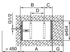
Sl. 2: Horizontalno postavljanje na zid
