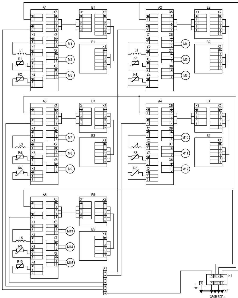
Схема индукционных плит комбо 700 и 900 серии, модели на 4 конфорки + однозонный гриль
