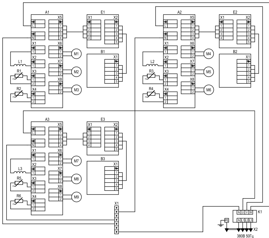
Схема индукционных плит комбо 700 и 900 серии, модели на 2 конфорки + однозонный гриль
