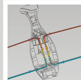
Система воздушного охлаждения
