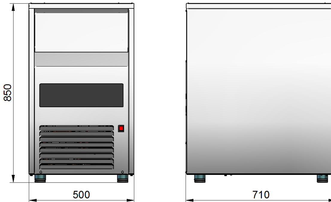
Рис. 1. Общий вид льдогенераторов ЛГ-60/20Г-01, ЛГ-60/20Г-02
