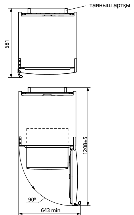
2 сурет – Тоңазытқыш (жоғарыдан көрініс)
