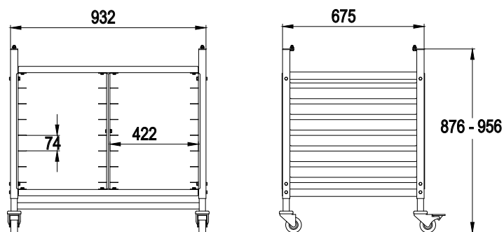
Размеры подставки с креплением для размещения продукции (в мм)
