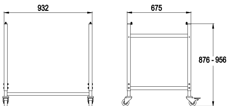
Размеры простой подставки (в мм)
