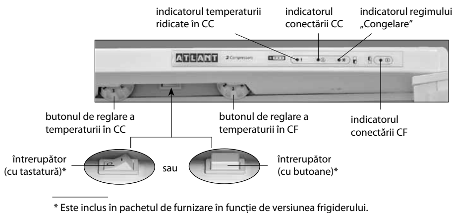
Figura 3 — Masca frigiderului
