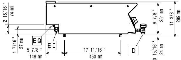
Вид сбоку
